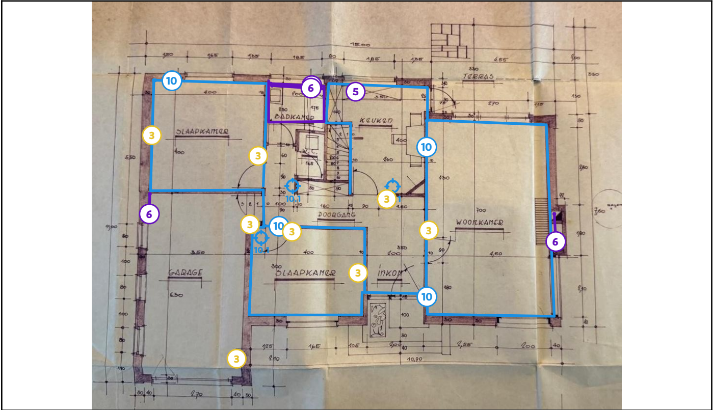
Legende van plan 1.3: +0 muren
